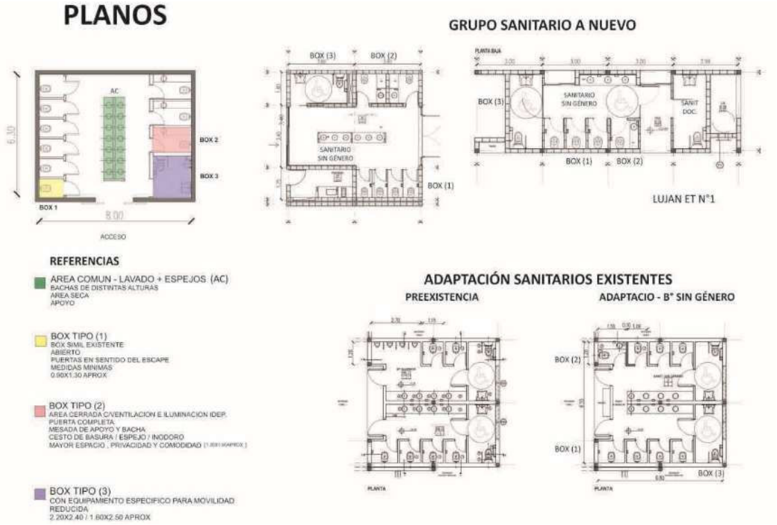
Figura 9: BAÑOS SIN GÉNERO - PLANOS
