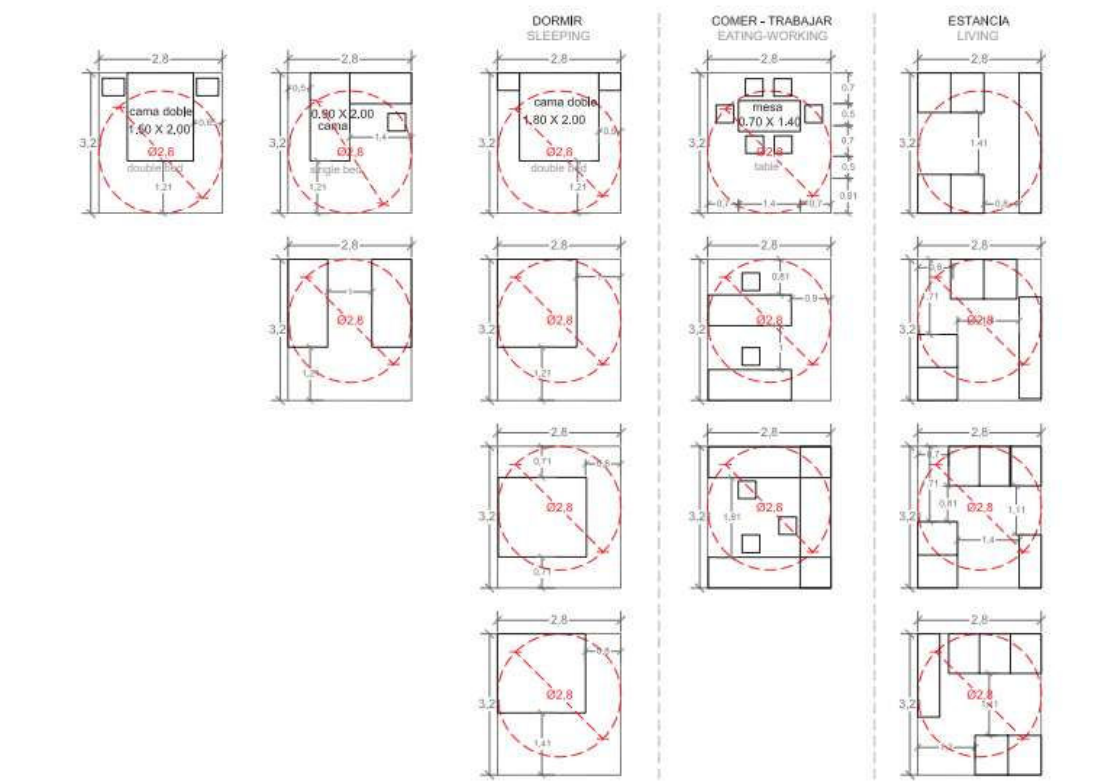
Figura 21: Estudio dimensional del espacio doméstico adaptable. Fuente: Herramientas para habitar el presente. La vivienda del siglo XXI Autores: Zaida Muxi, Josep M. Montaner, David H. Falagán 2010-2011
