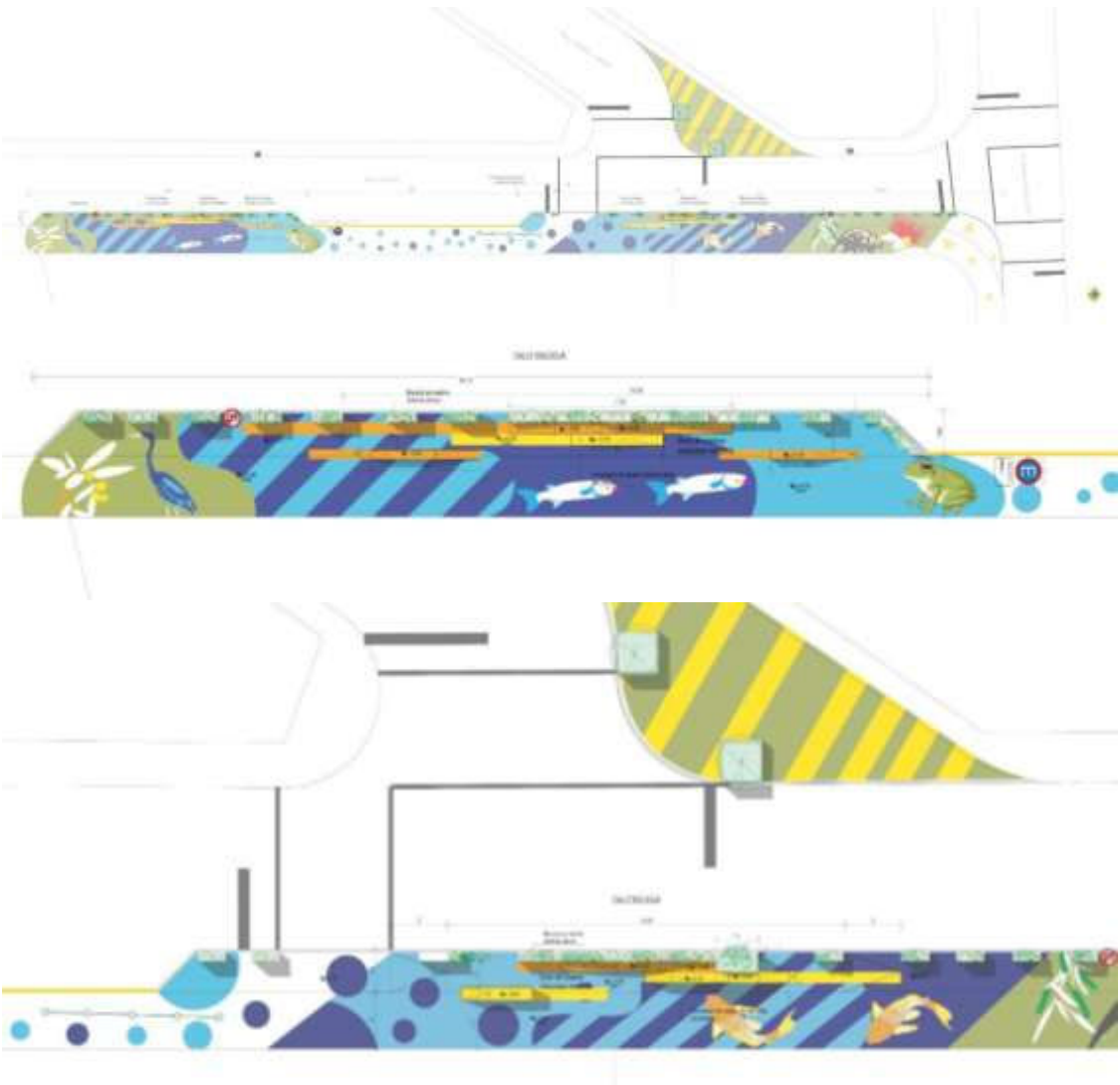
Figura 9: Anteproyecto escuela n.º 42. Fuente: elaboración propia equipo LUPA, 2023.
