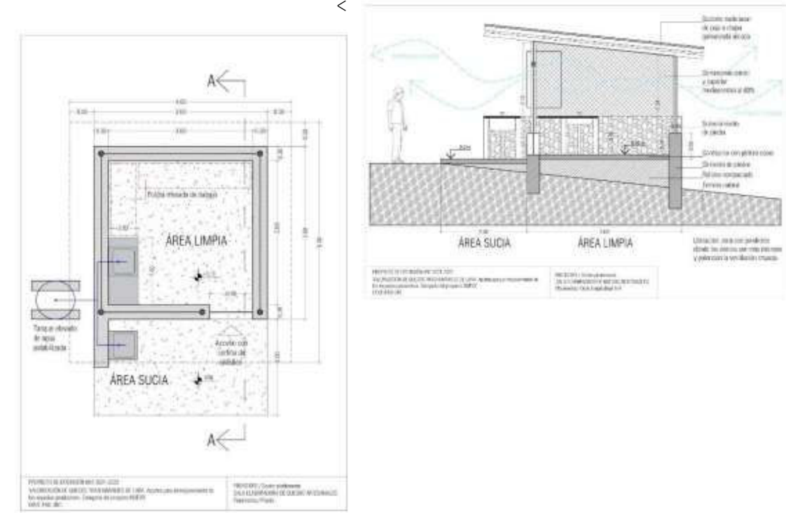
Figura 4. Planimetría de Sala Elaboradora de quesos para "La Costa" (piedemonte de la serranía), construcción finalizada en Puesto de Dina y Braulio. Fuente: Elaboración propia en el marco del P. de Ext. 2022 UNT.
