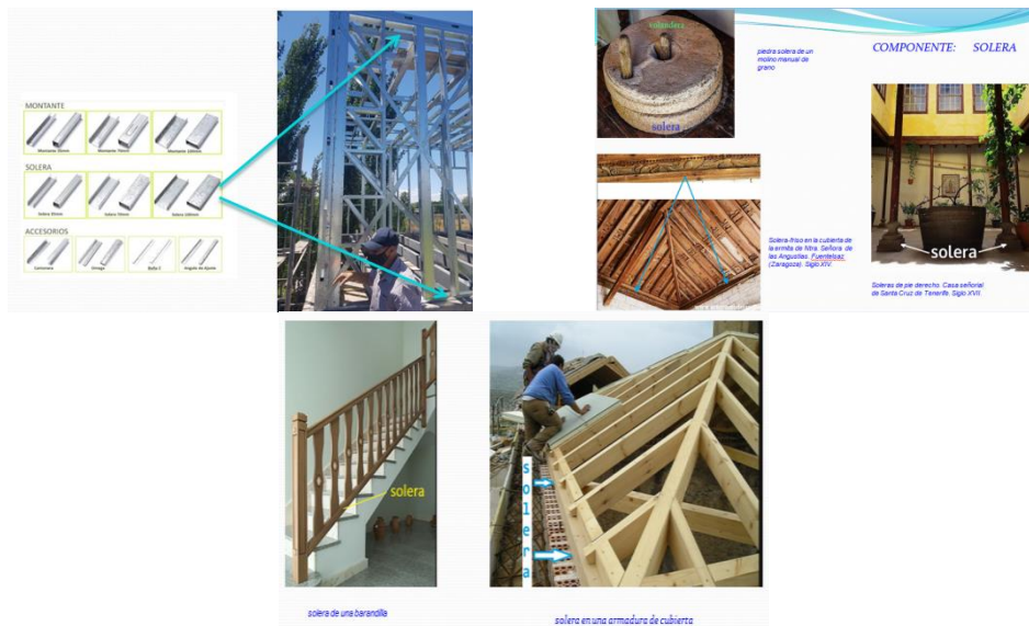
Figura 2: Ejemplo donde el término solera tiene distintos significados, posiciones en obra, materiales y usos entre otros
