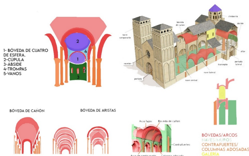
Figura 4: Análisis del espacio interior de una catedral románica
