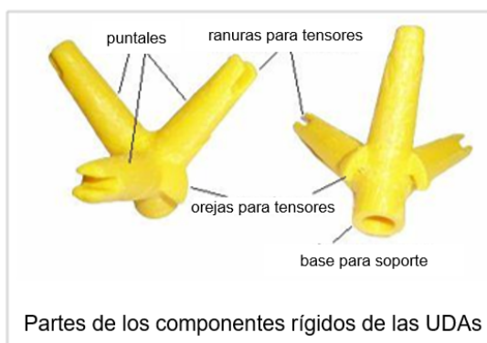
Figura 3: Prototipos de componentes rígidos de las UDAs, impresos en 3D
