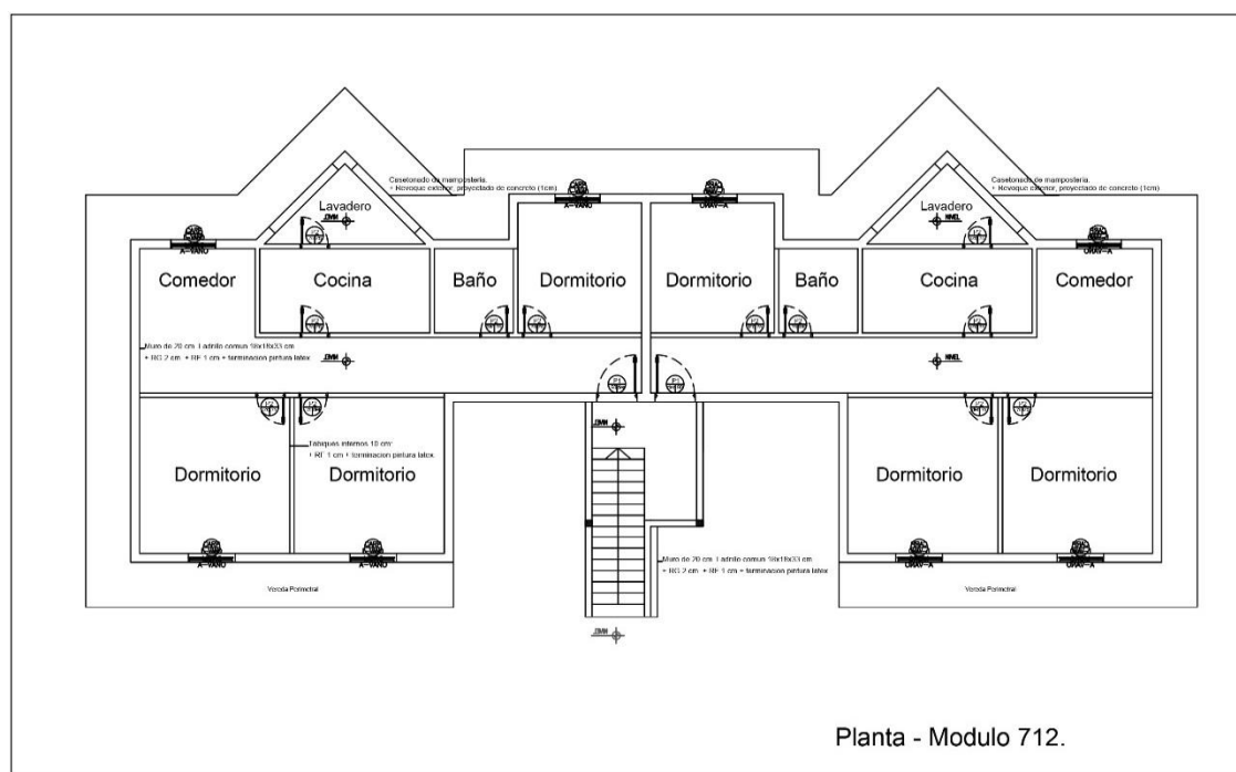
Figura 2. Planta de dos unidades tipo del Barrio Catonas. Dibujo: Tomás Rougier.
