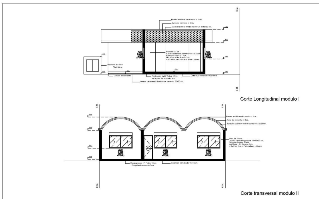
Figura 1. Cortes del Barrio PAMI. Dibujo: Tomás Rougier.
