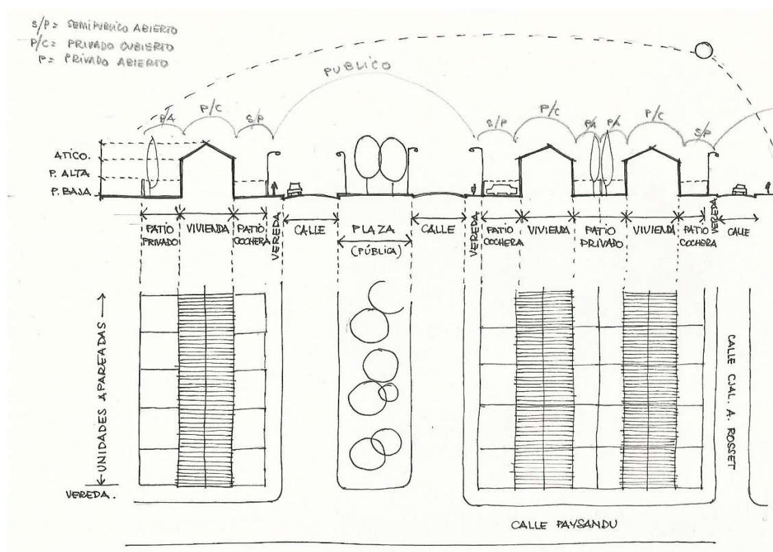
Figura 3. Corte general del Barrio Arquitectura. Dibujo: Rafael Indart.
