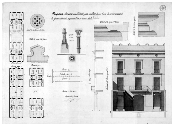
Figura 6: Proyecto de fachada para patio de una casa de un rico comerciante. Alumno: Cayetano Miret Reventos. Escuela de maestros de obras y agrimensores (1867). AG000410. Fuente: Dossier Càtedra Gaudí (ETSAB). Recuperado de: https://catedragaudi.upc.edu/ca/fons/2.Fondoesuelasymaestrosdeobras.pdf/view
