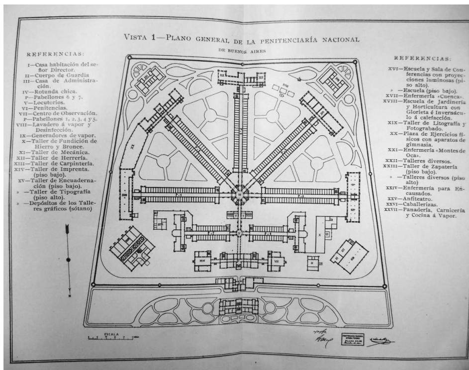
Figura 3: Plano de la Penitenciaría Nacional de Buenos Aires. Fuente: Ballve, 1907.
