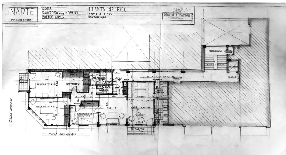
Figura 5: Anteproyecto de edificio de viviendas en altura, esquina de Moreno y Saavedra, ciudad de Buenos Aires (1963). Planta del cuarto piso. Repositorio: Colección José Manuel Felipe Pastor, Archivo Documental del IAA, FADU, UBA.
