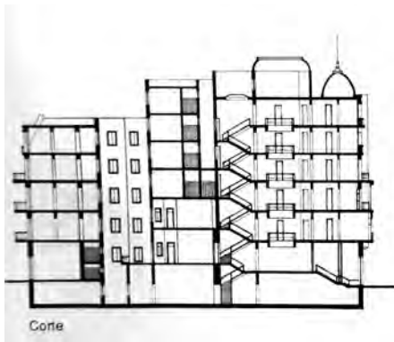
Figura 7: Palacio Vera. Corte, Plata Tipo y Planta Baja. Fuente: Solsona, J. y Hunter, C., 1990, La Avenida de Mayo. Un proyecto Inconcluso . p. 116. Buenos Aires, Argentina: FADU.
