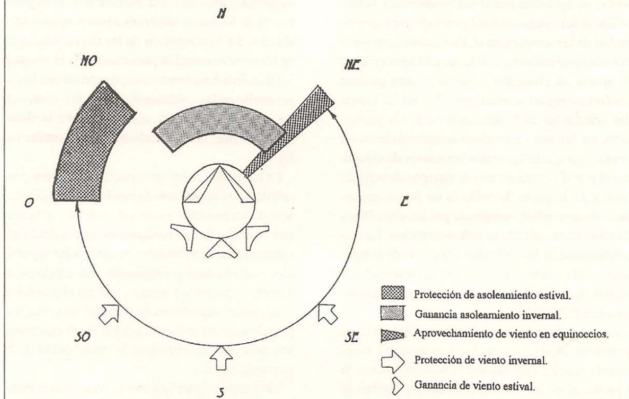
Figura 4: Variables de asoleamiento e impacto de viento en función de la orientación.
