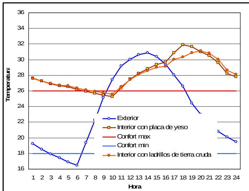
Figura 3. Simulación de la temperatura interior en invierno, con muros interiores de placa de yeso o ladrillo de tierra cruda.
