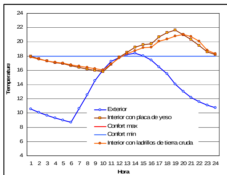
Figura 2. Simulación de la temperatura interior en invierno, con muros interiores de placa de yeso o ladrillo de tierra cruda.
