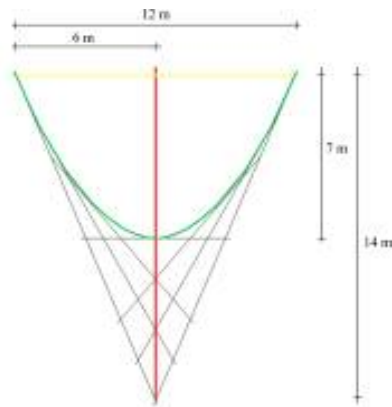
Figura 9: Construcción parábola. Polígono funicular
