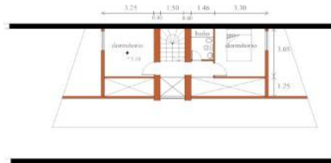
Figura 4: Planta alta
