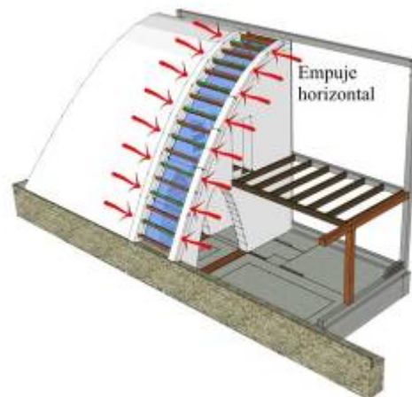
Figura 14: Empujes horizontales en la raja
