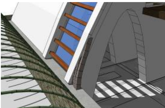
Figura 15: Sobrecimiento: canaleta, apoyo bóveda y pérgola
