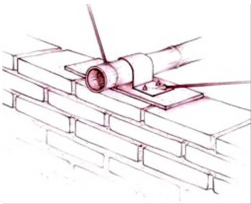
Figura 6. Amarre de los tensores del techo a los muros.
