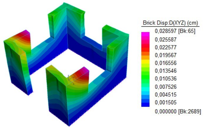
Figura 9. Casa de la prueba de PUCP
