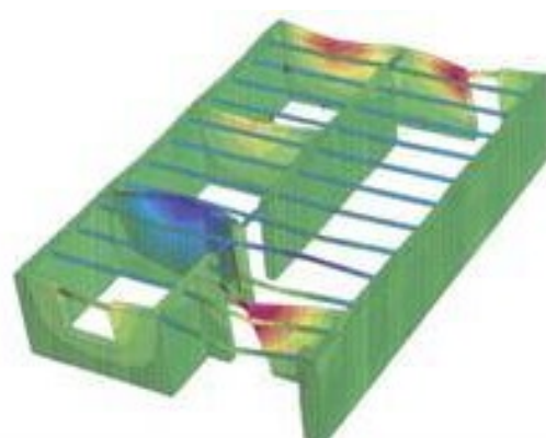
Figura 7. Análisis dinámico, mecanismo de colapso.
