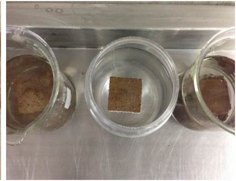
Figura 6. Probeta desintegrada a la izquierda, a la derecha la de tierra compactada y al centro se mantiene íntegra la probeta de tierra estabilizada y compactada. Laboratorio de Materiales de la UAM-Xochimilco.
